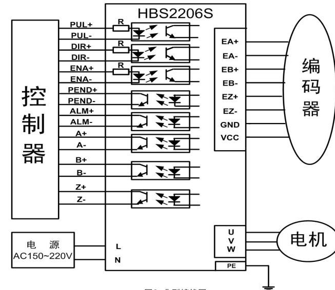
图6 典型接线图
