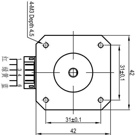
外形图 DIMENSIONS unit: mm
